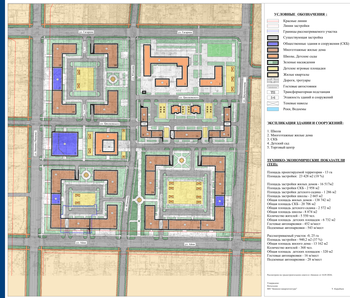
Проект застройки ограниченный улицами: ул. Бакаева, ул. Айни, ул. Джунусалиева, ул. Гагарина в городе Бишкек (1-этап) Генеральный план
