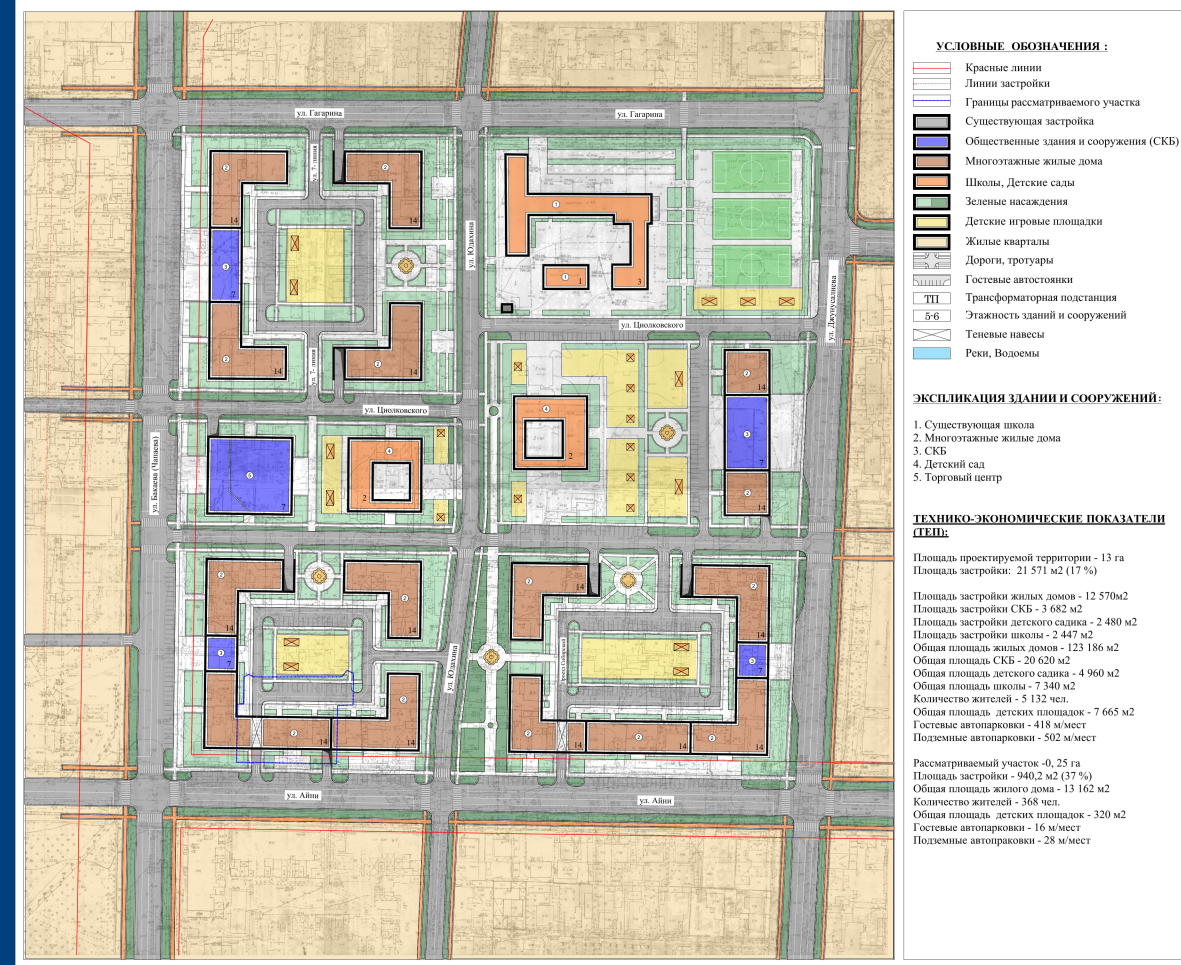
Проект застройки ограниченный улицами: ул. Бакаева, ул. Айни, ул. Джунусалиева, ул. Гагарина в городе Бишкек (1-этап) Генеральный план
