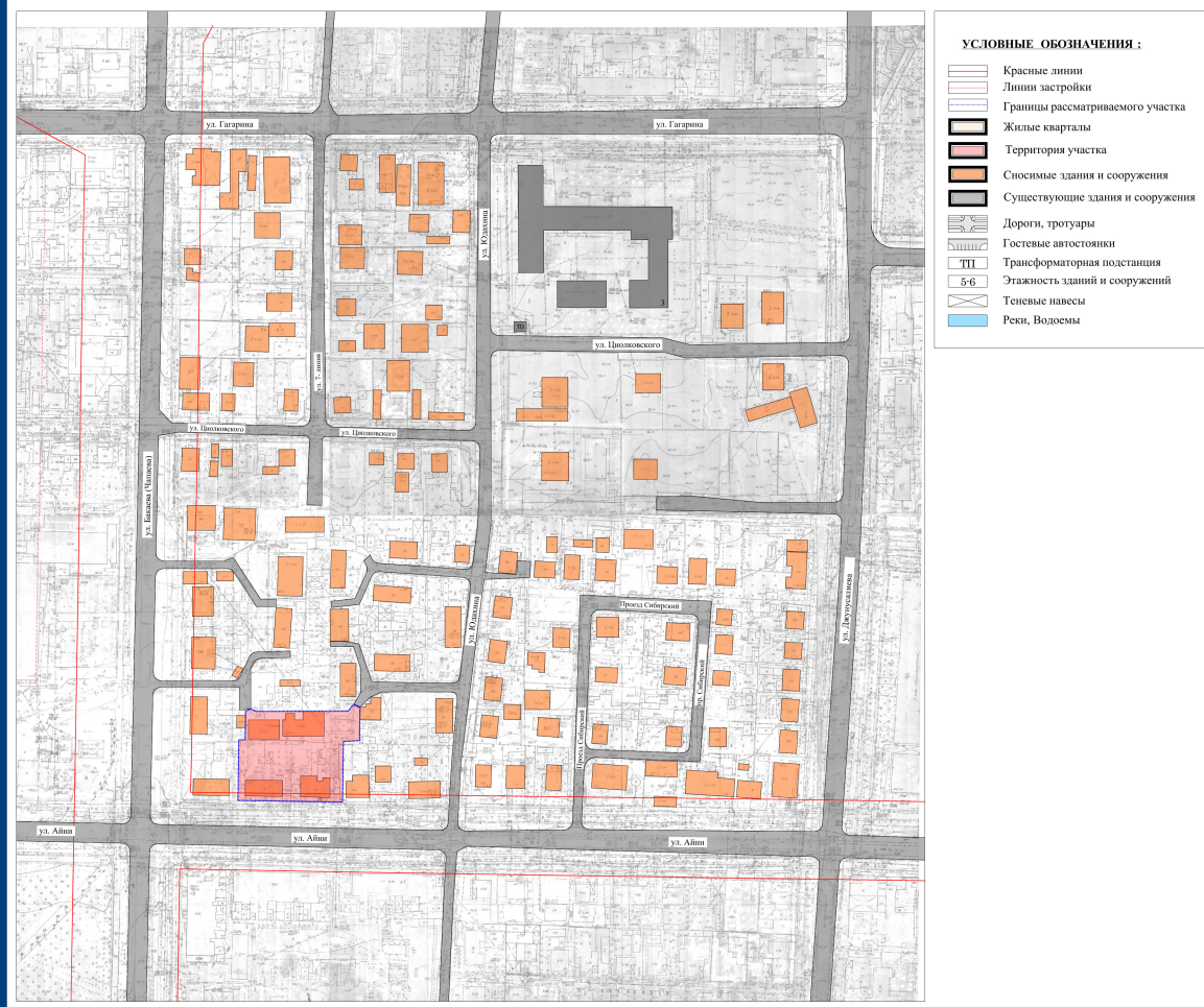
Проект застройки ограниченный улицами: ул. Бакаева, ул. Айни, ул. Джунусалиева, ул. Гагарина в городе Бишкек (1-этап) Опорный план
