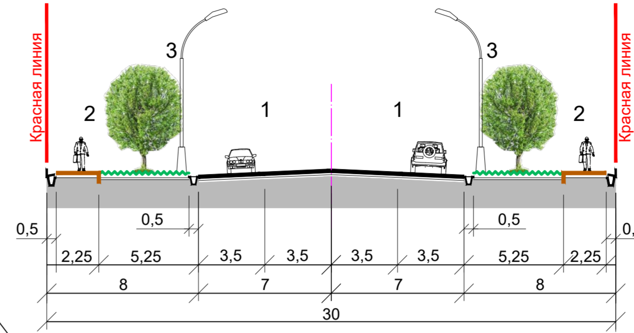
Масштаб 1:200 (размеры всех элементов даны в метрах) 1- проезжая часть; 2- тротуары; 3- полосы озеленения.
