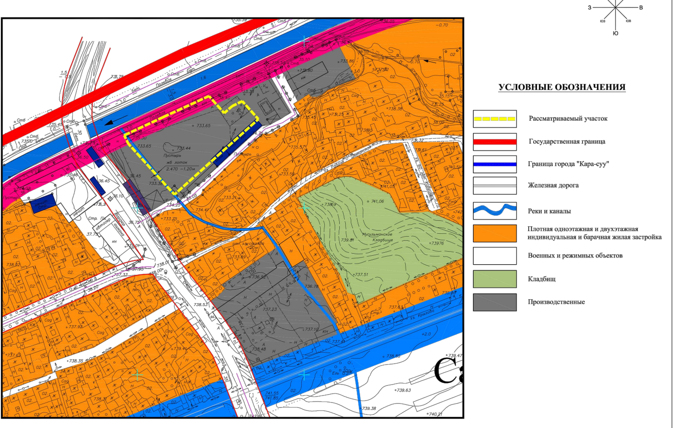
Генеральный план г. Кара-Суу
