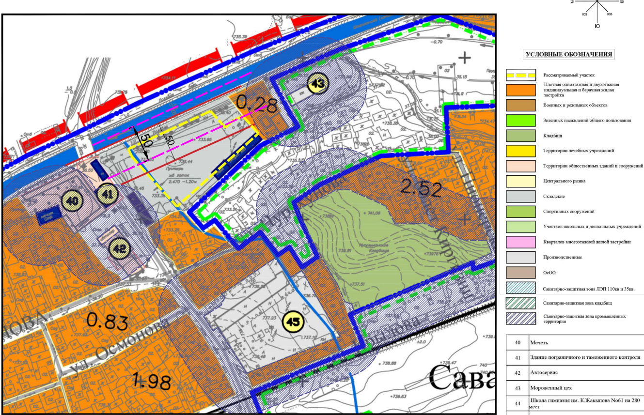
Опорный план г. Кара-Суу
